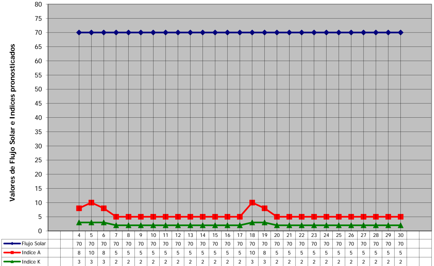
Flujo Solar Indice A Indice K
