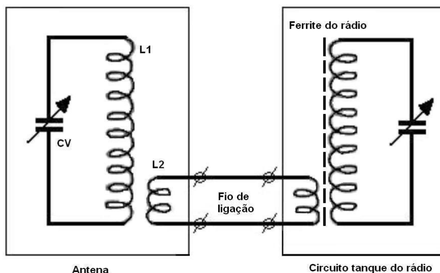
Esquema usado para o acoplamento da antena no rádio
